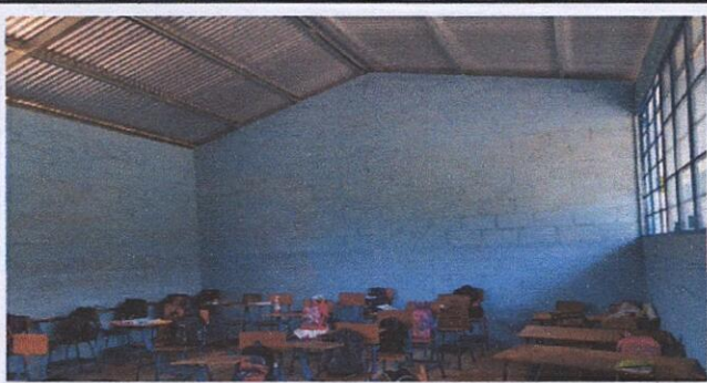
Foto 3: Colocación y soldadura de vigas, costaneras.Colocación de cubierta de lamina de zinc .
